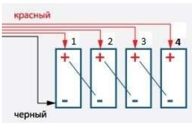
Аккумуляторы 2 В №№ 1÷4
